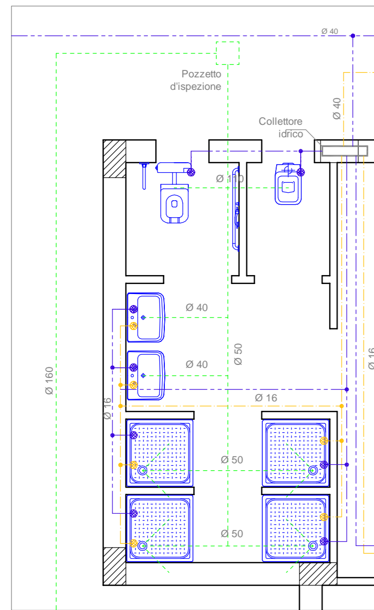
PARTICOLARE IMPIANTI Scala 1:50
