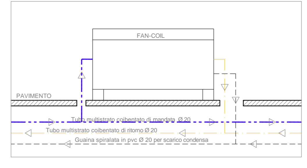
PARTICOLARE COLLEGAMENTO RETE fan-coil Scala 1:20
